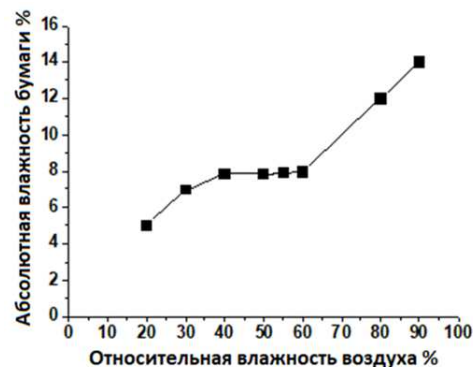
Рис. 1. Зависимость влажности бумаги от относительной влажности (рисунок из http://www.arzpuck.ru/arz121.html ).
