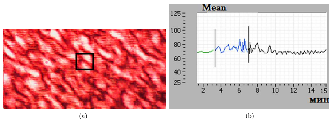
Рис. 10. Влияние ладони человека на картину спеклов при герметичной изоляции от окружающей среды черной бумаги датчика “Спеклоскопа” тефлоновой пленкой. (а) – спекл-картина, квадратом показана область, для которой рассчитывалась интенсивность ее свечения; (б) – Вертикальными линиями показаны моменты приближения и удаления ладони человека к датчику “Спеклоскопа”. Ладонь ставилась на подставку, которая обеспечивала расстояние от ладони до датчика, покрытой тефлоном в 7-10 мм.
