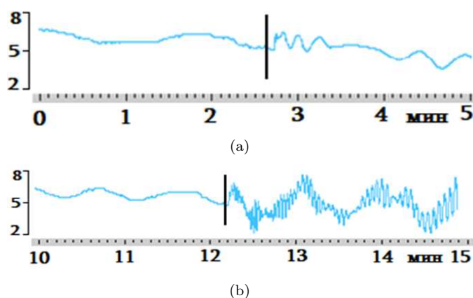
Рис. 5. Влияние герметично изолированной тефлоном капли воды на показания "Биоскопа". (а) – Сигналы "Биоскопа" при приближении к его датчику "тефлоновой" камеры без воды. (б) – Сигналы "Биоскопа" при приближении к его датчику "тефлоновой" камеры с каплей воды. Линией отмечен момент приближения камеры к датчику "Биоскопа".
