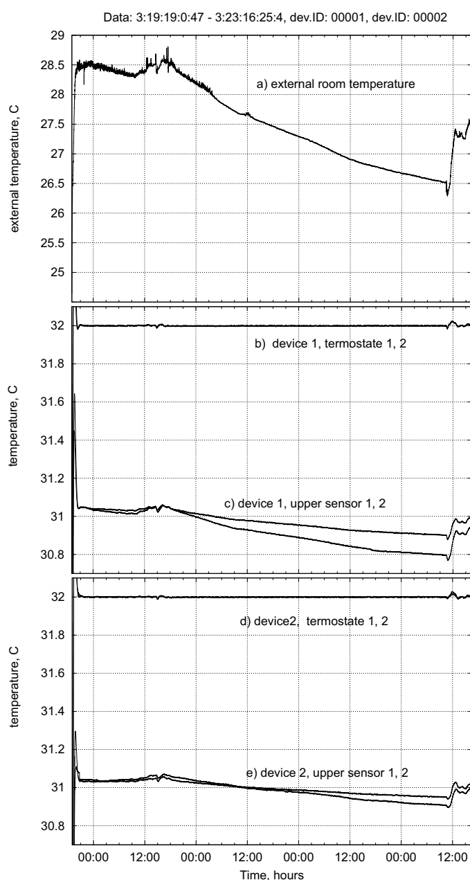
Рис. 3. Сравнение температурных данных: а) внешняя температура в лаборатории, б) и д) термостаты устройства 1 и 2; в) и е) сенсоры, расположенные на верхнем конце термоконтейнера (вне термостата) устройства 1 и 2.
