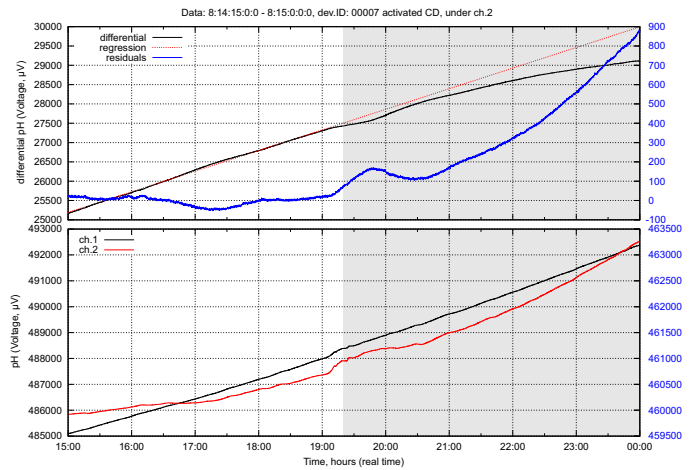
Рис. 9. Эксперимент 15.08.2015, иллюстрация применения регрессионного анализа для pH кривых, см текст. На нижнем графике представлены исходные pH_1, pH_2 кривые первого и второго каналов, черная кривая на верхнем графике – дифференциальная кривая dpH = pH_1 - pH_2 , которая аппроксимируется линейной функцией f(x) на участке фоновой динамики. Значения остатка dpH - f(x) показаны синей кривой на верхнем графике. Серой полосой показана область воздействия (CD диск под каналом 2).
