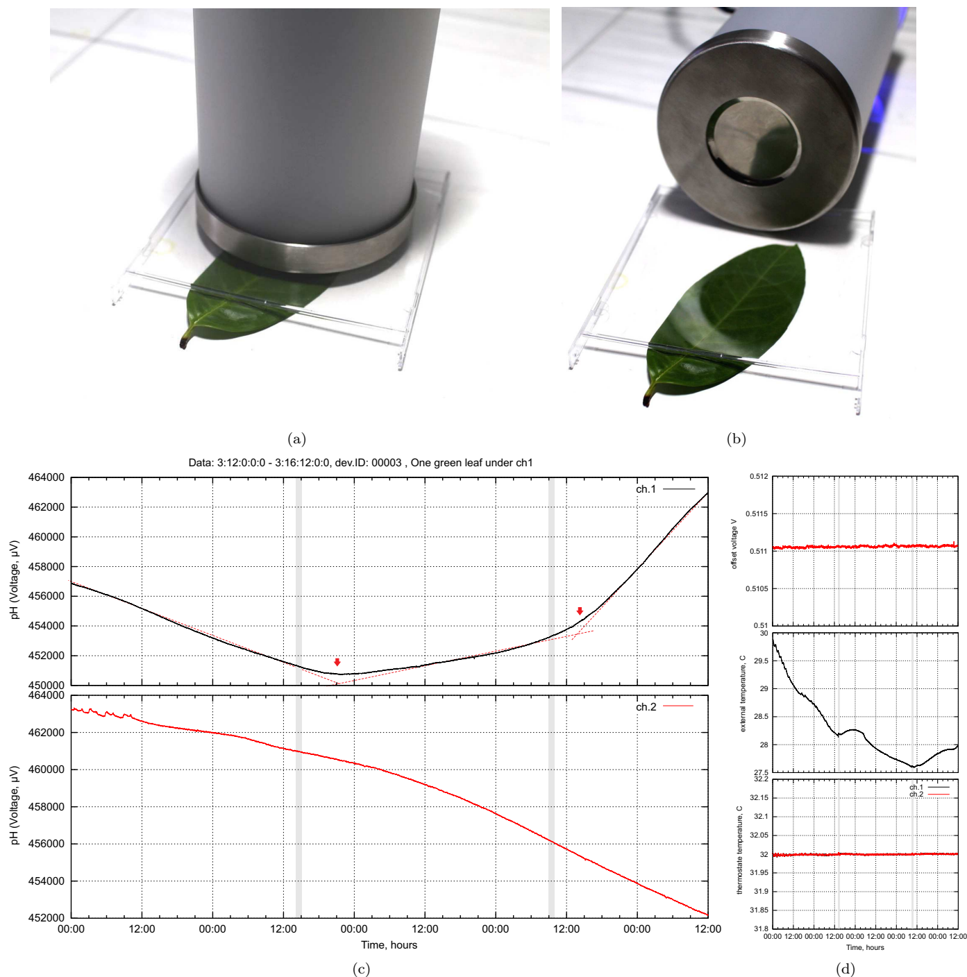
Рис. 14. Пример эксперимента по воздействию сорванного зеленого листа на динамику pH питьевой воды (10мл контейнеры в металлическом термостате), pH электроды Hanna Instruments HI1131B, измерительный прибор CybRes dpH 3.0. Лист находится под каналом 1. (а) Внешний вид термостата с pH электродом и контейнером с водой, канал 1; (б) Металлическое дно термостата; (с) Динамика pH значений обоих каналов, напряжение смещения 0.511В; (д) Динамика некоторых вспомогательных данных: напряжение смещения, внешняя температура в лаборатории, температура термостатов с pH электродами и контейнерами с водой. Первая серая полоса показывает размещение зеленого листа под термостат канала 1, вторая серая полоса отмечает удаление листа из-под термостата. Отчетливо видно изменение тренда pH канала 1 через 4-5 часов после размещения/удаления зеленого листа. Данные из температурных, ЭМ, акселерометров и других сенсоров указывают на то, что тепловой, механический и электромагнитный пути переноса взаимодействия в этом эксперименте не играют существенной роли.
