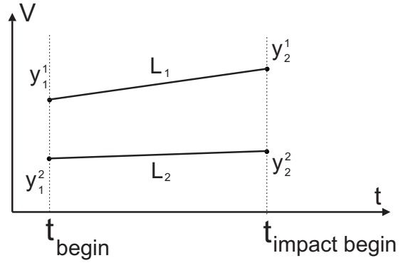
Рис. 8. Иллюстрация для расчета коэффициентов \alpha, \beta при одноканальном ЛКП.
