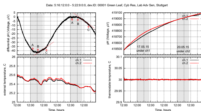
Рис. 16. Сравнение динамики каналов прибора N1 в эксперименте 17.05.15 и 20.05.15. Совмещение динамики pH каналов производилось методом ЛКП.
