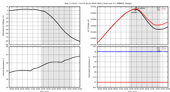
Рис. 12. Иллюстрация эффекта связанных измерительных жидкостей, серой полосой показано воздействие (свежесрезанный зеленый лист под каналом 1).
