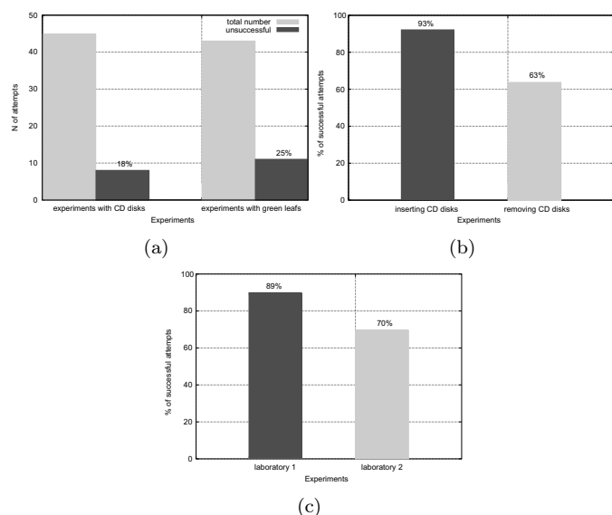
Рис. 15. Анализ результатов экспериментов с CD дисками и зелеными листьями. (a) Соотношение общего числа экспериментов к числу экспериментов с отрицательным результатом; (b) Процентное соотношение экспериментов с позитивным результатом при внесении диска в систему и при выносе диска из системы; (c) Процентное соотношение экспериментов с позитивным результатом в помещениях 1 и 2.
